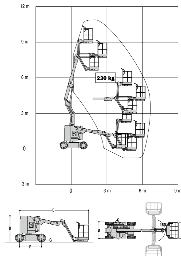
JLG Model E300AJP
